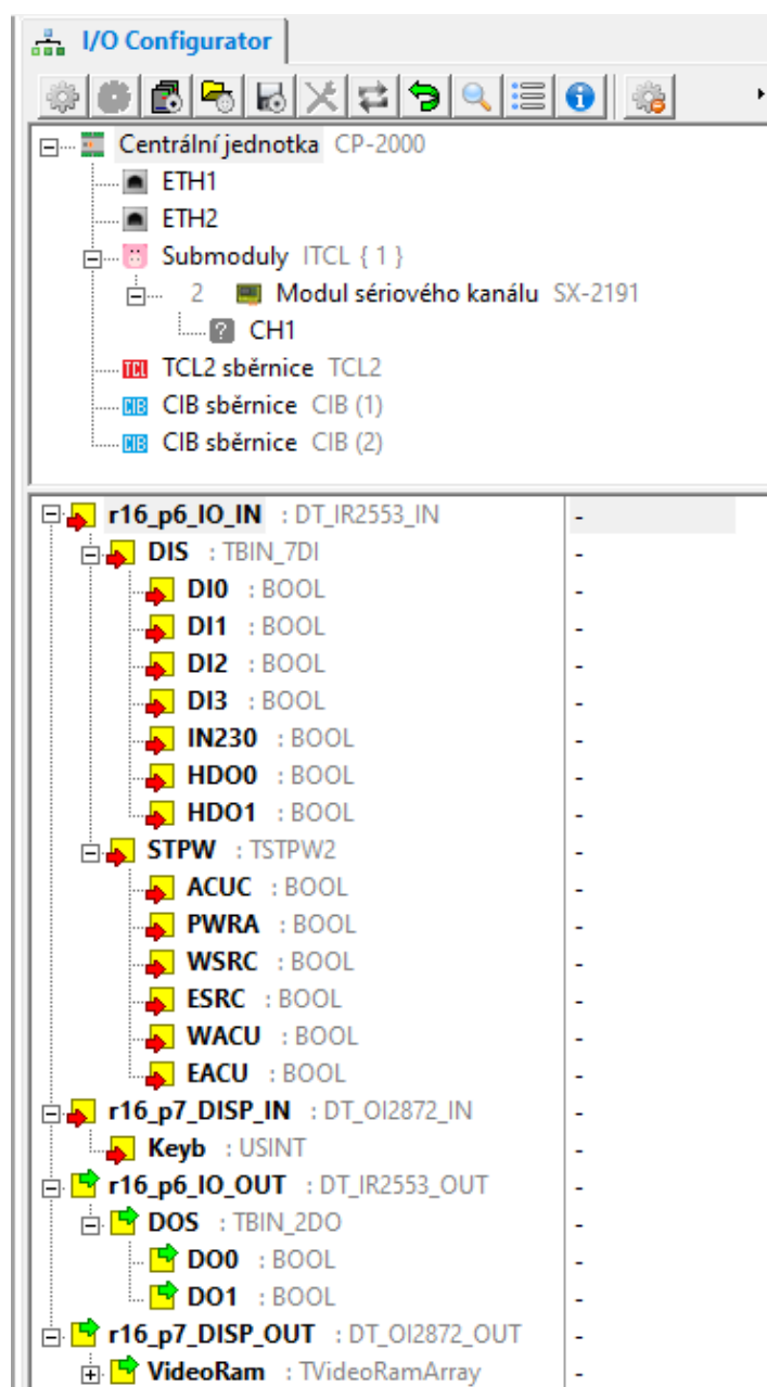
Obr.7.2 Okno nástroje I/O Configurator
