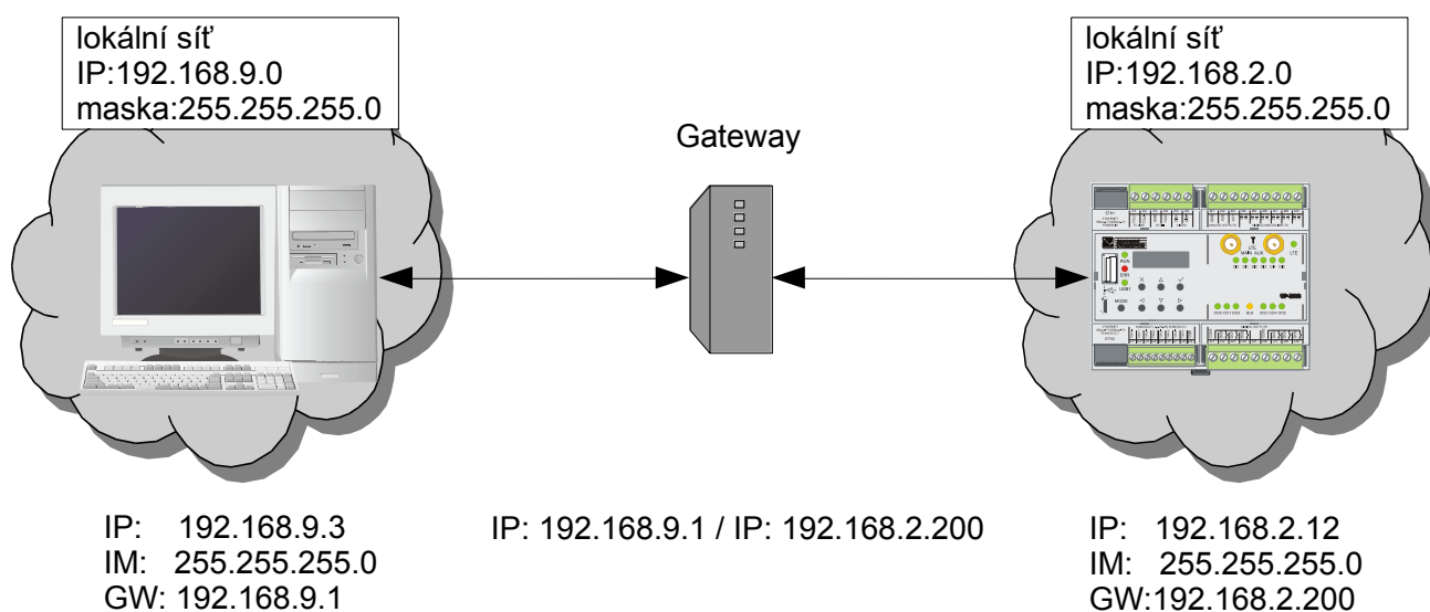
Obr.7.8 Příklad propojení dvou sítí pomocí brány (gateway)
