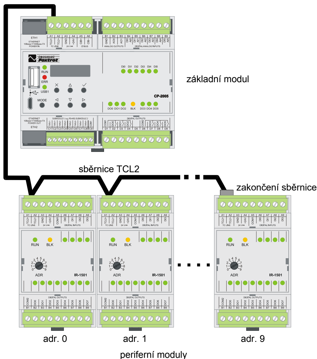
Obr.1.3 Příklad sestavy PLC TECOMAT FOXTROT 2 s jednou sběrní TCL2
