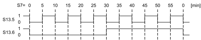
Stav bitových proměnných %S13 ve vztahu k minutovému čítači %S7
