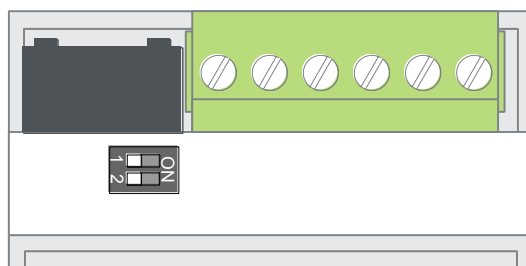
Obr.9.1 Umístění DIP přepínačů 1 a 2 pod štítkem u konektoru ETH1 a svorkovnice A, přepínače jsou nastavené pro běžný provoz
