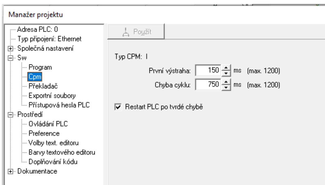
Obr.7.9 Nastavení konfiguračních konstant
