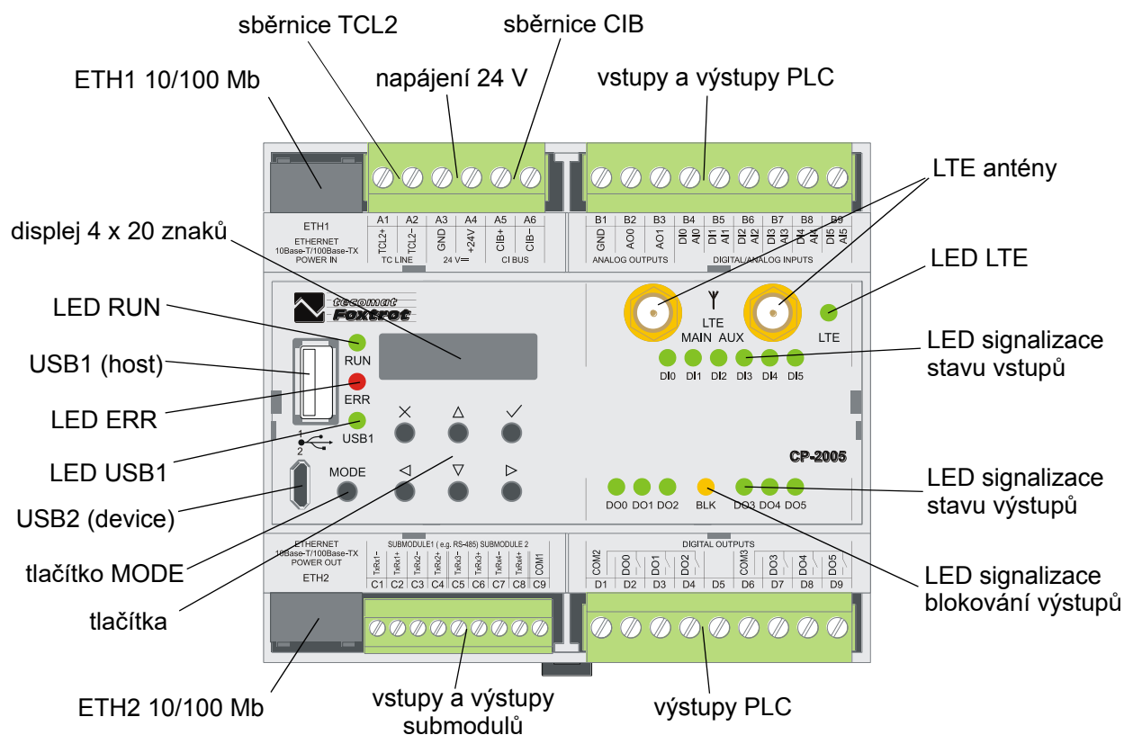
Obr.2.2 Základní modul PLC TECOMAT FOXTROT 2 šířky 6M (CP-2005 s rozhraním LTE1)
