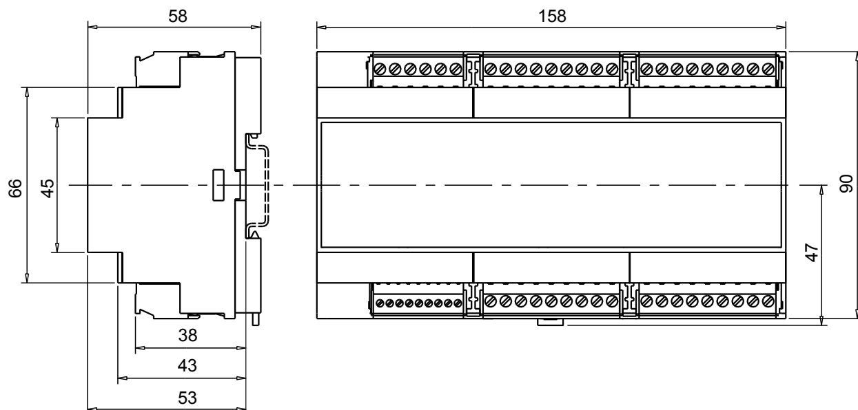
Obr.1.6 Rozměry základních modulů CP-2000, CP-2007
