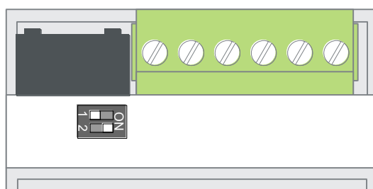
Obr.9.2 Nastavení DIP přepínačů 1 a 2 v režimu pro tovární nastavení
