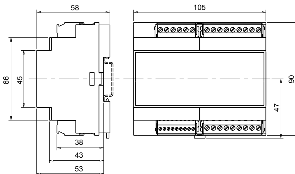
Obr.1.5 Rozměry základních modulů CP-2005, CP-2080
