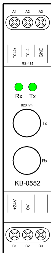
Obr.4.1 Modul optického propojení KB-0552
