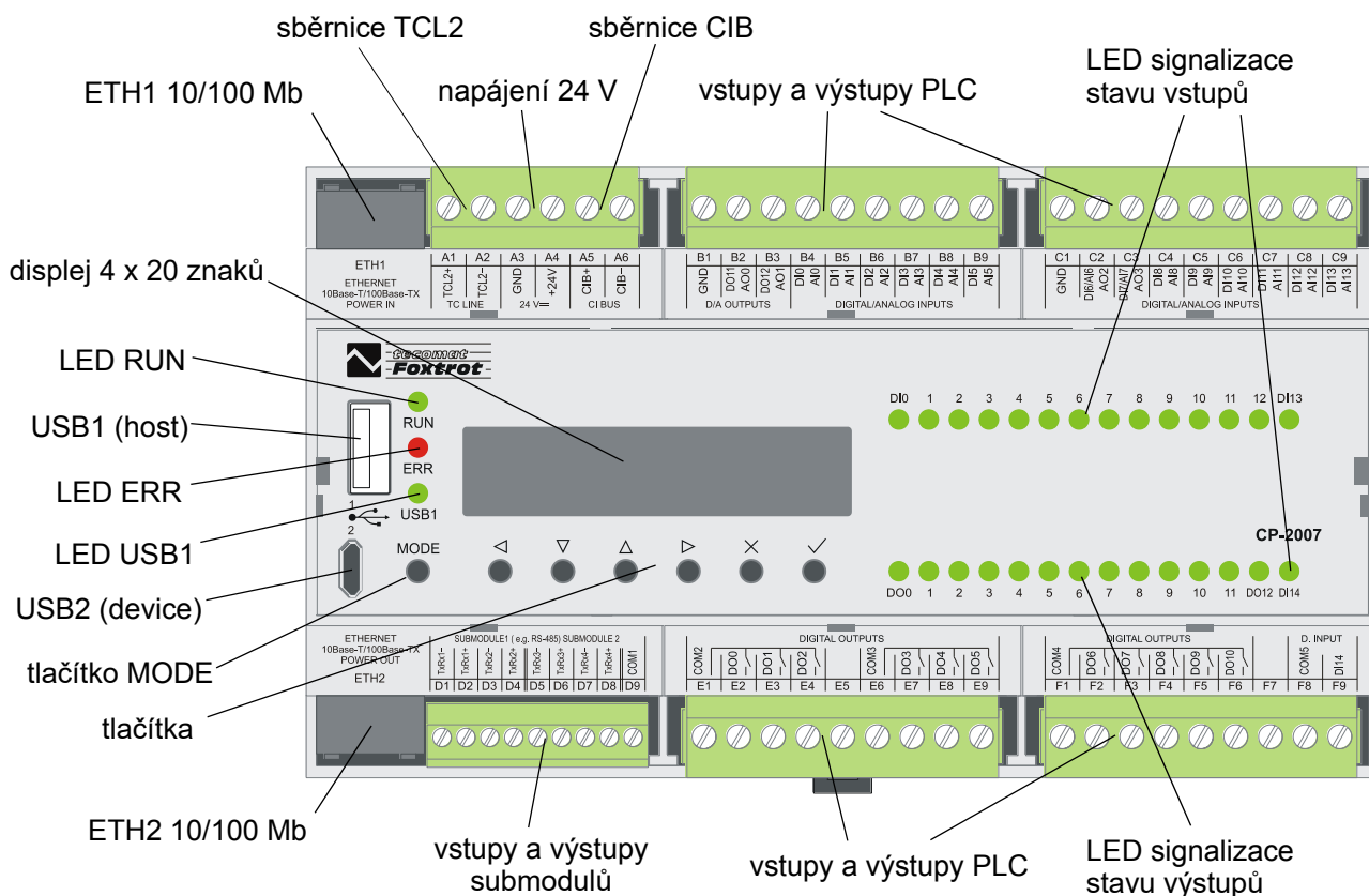
Obr.2.3 Základní modul PLC TECOMAT FOXTROT 2 šířky 9M (CP-2007)
