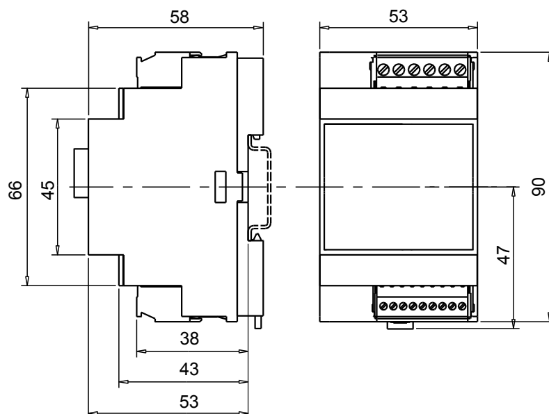
Obr.1.4 Rozměry základního modulu CP-2090
