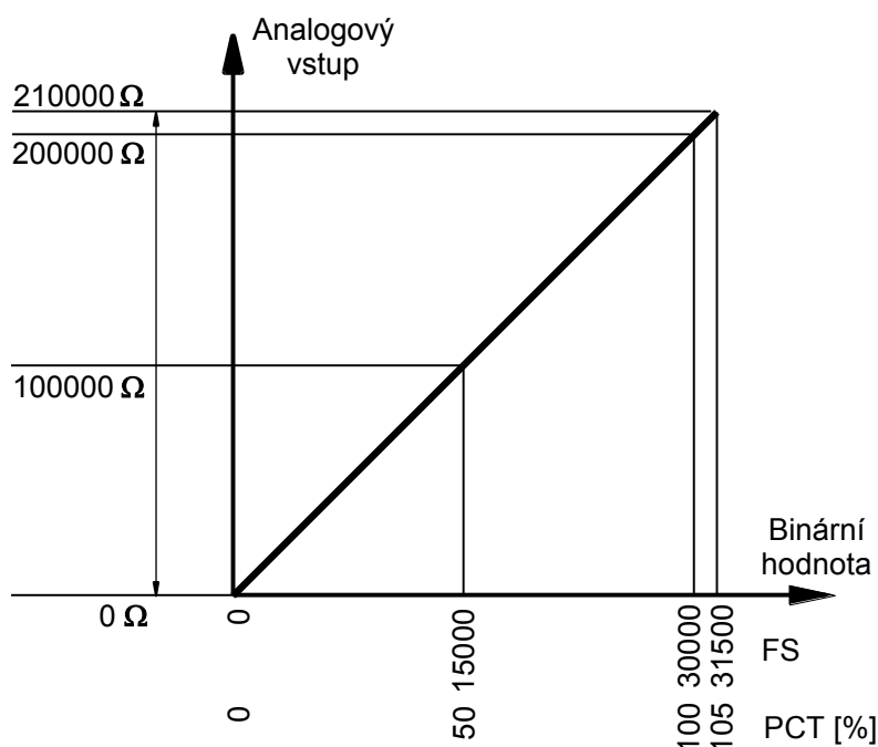
Obr.5.14 Odporový rozsah do 200 k \Omega analogových vstupů
