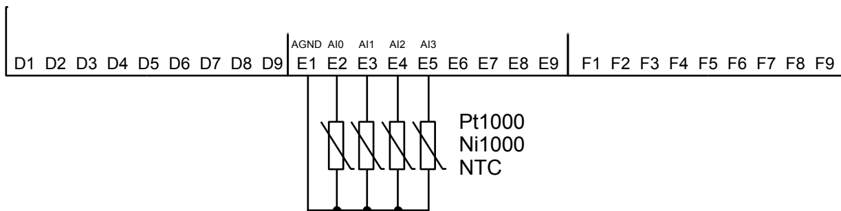
Obr.4.3 Typický příklad připojení signálů k analogovým vstupům
