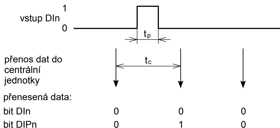
Obr.5.10 Funkce detekce krátkých pulzů do log.1 t_p - šířka pulzu, t_c = doba cyklu PLC
