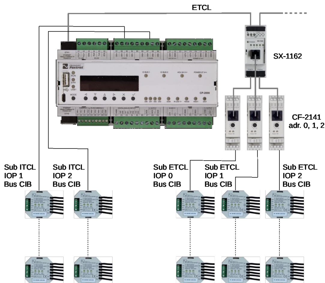
Obr.3.2 Příklad sestavy s pěti linkami CIB
