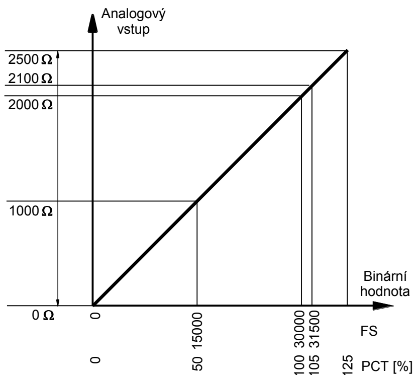
Obr.5.13 Odporový rozsah 2 k \Omega analogových vstupů
