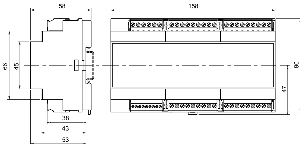
Obr.2.1 Rozměry základních modulů CP-2000
