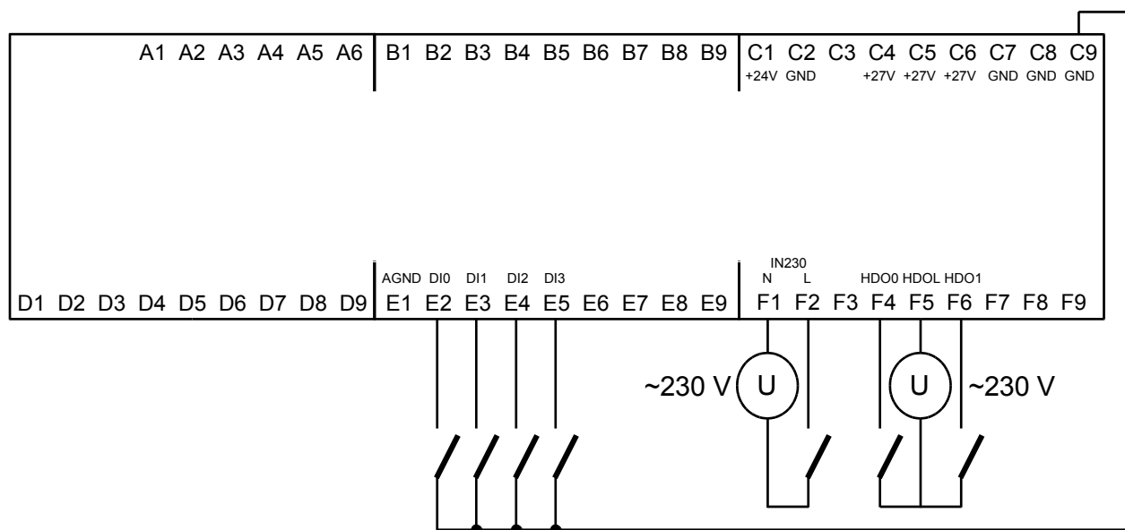
Obr.4.1 Typický příklad připojení spínačů k binárním vstupům
