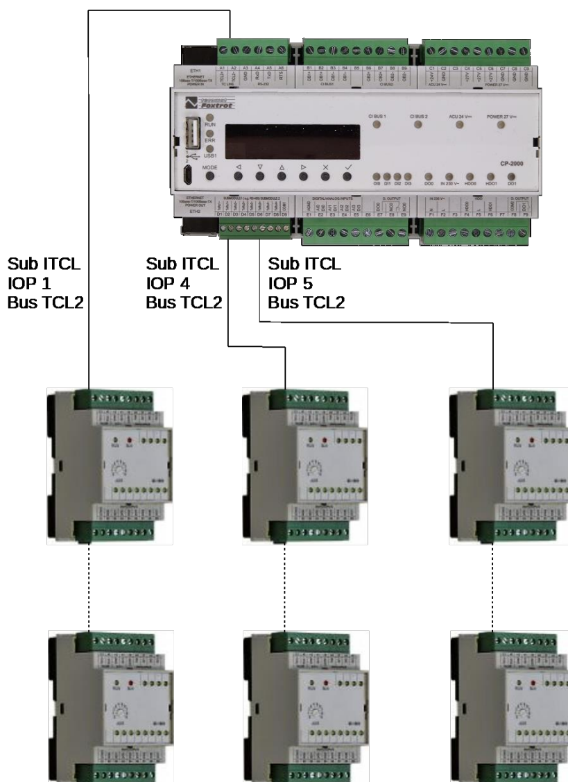
Obr.3.1 Příklad sestavy se třemi sběrnicemi TCL2
