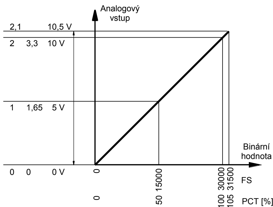
Obr.5.11 Napěťové rozsahy analogových vstupů
