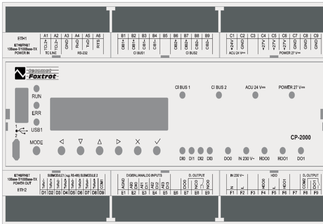
Obr. 4.1 Zapojení binárních a analogových vstupů / výstupů základního modulu CP-2000
