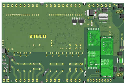
Obr. 7.1 Umístění výměnných submodulů s rozhraním sériového kanálu na spodní desce základního modulu CP-2000
